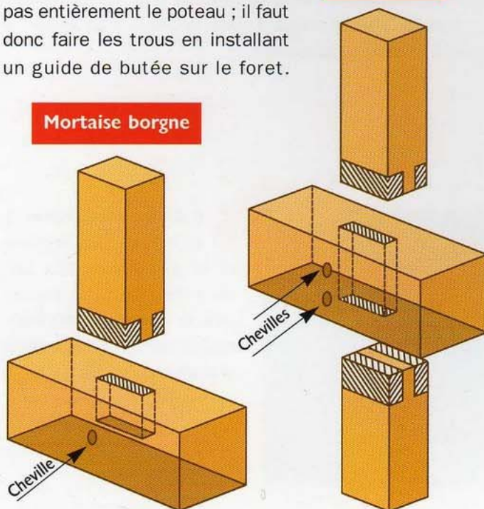
Mortaise traversante
